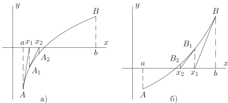
Рис. 4.14 Метод касательных
