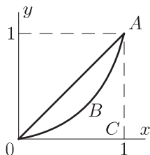
Рис. 6.4 Кривая Лоренца
