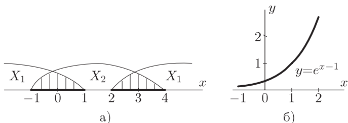
Рис. 1.10
