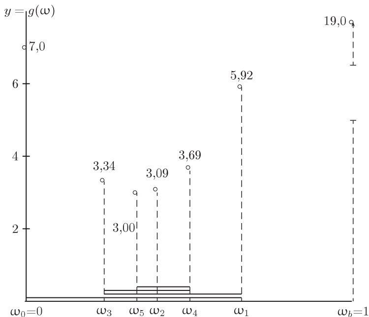
Рис. 4.12 Итерации метода золотого сечения
