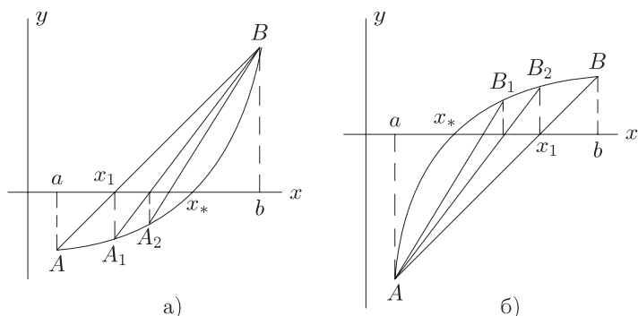
Рис. 4.13 Метод хорд
