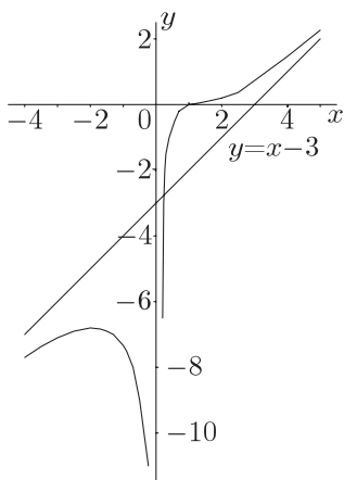
Рис. 4.9 График функции
