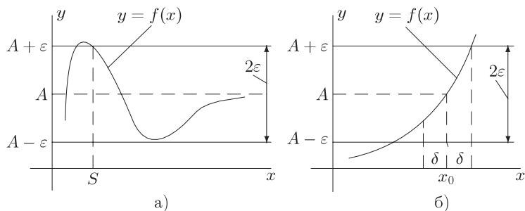
Рис. 2.1 Предел функции
