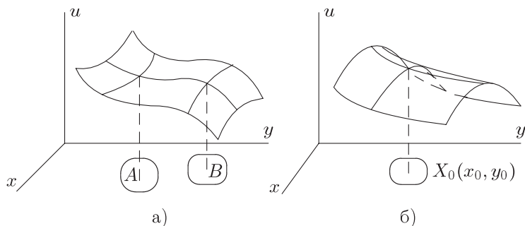
Рис. 5.6
