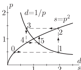
Рис. 1.7 Паутинная модель
