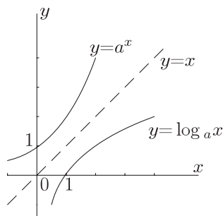
Рис. 1.3 Обратные функции
