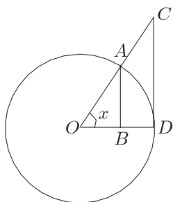
Рис. 2.3 Первый замечательный предел
