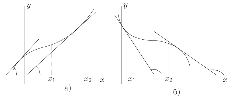
Рис. 4.2 Возрастание и убывание функции
