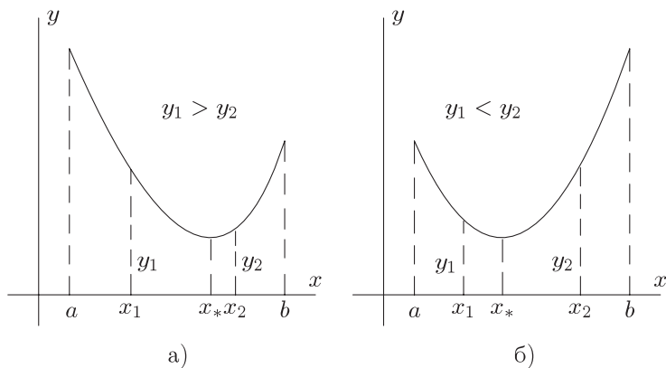
Рис. 4.10 К методу исключения интервалов
