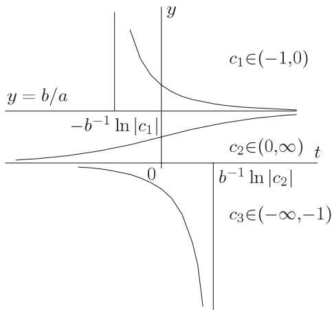
Рис. 7.2 Интегральные кривые
