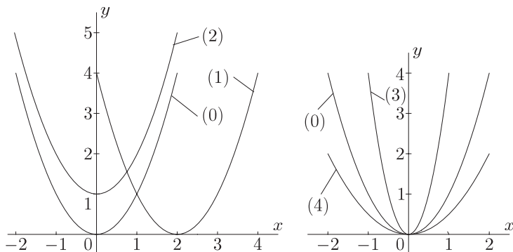
Рис. 1.4 Преобразование графиков
