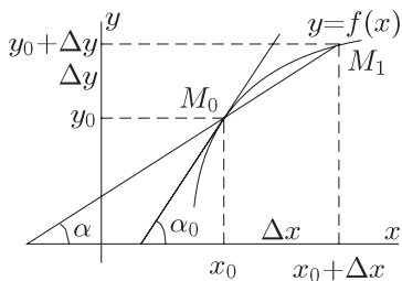
Рис. 3.1
