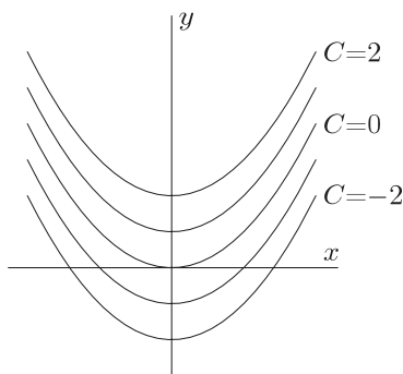
Рис. 7.1 Интегральные кривые
