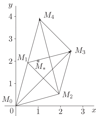
Рис. 5.8 Симплексный метод
