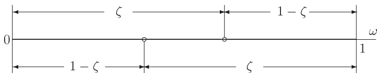
Рис. 4.11 Метод золотого сечения
