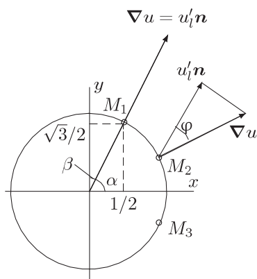
Рис. 5.4 Производная по направлению и градиент
