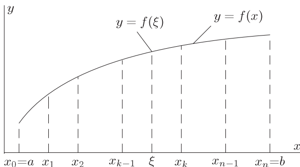
Рис. 6.1 Интегральная сумма
