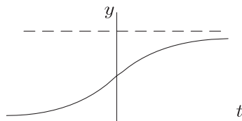
Рис. 7.6 Логистическая кривая
